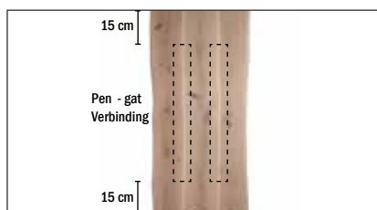
3 Lamellen / Planken
